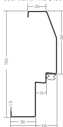
door frame PM84/150
