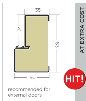
frame Termo ODS56
