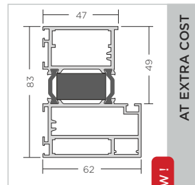
frame Termo ALU 68
