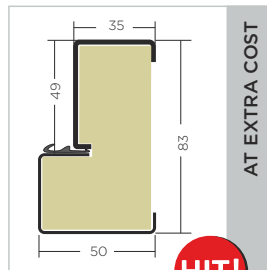
frame Termo ODS68
