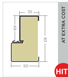
frame Termo ODS68
