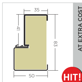
frame Termo ODS56
