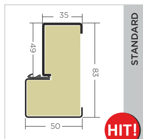
frame Termo ODS68
