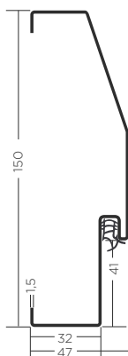
door frame PD56/150
